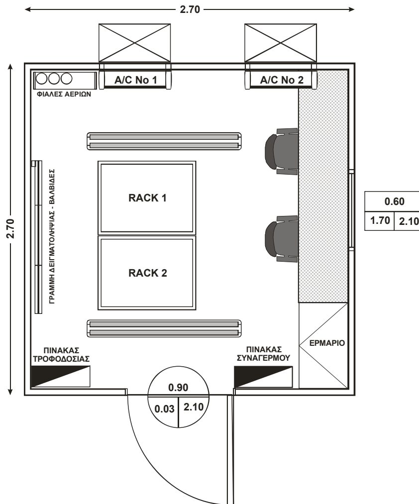
Κάτοψη Κλωβού
